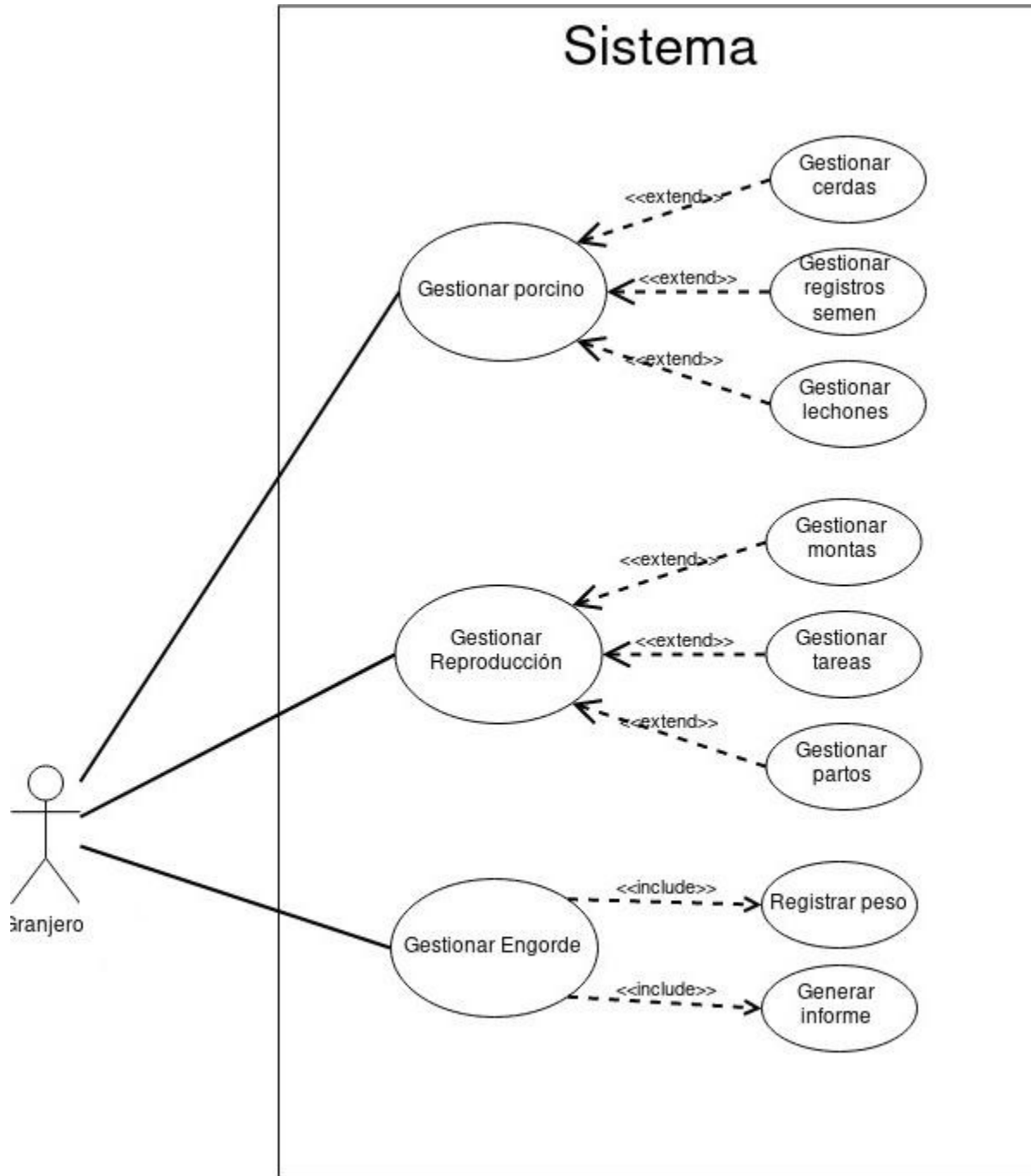
Figura 2. Diagrama de Casos de uso Menú principal
