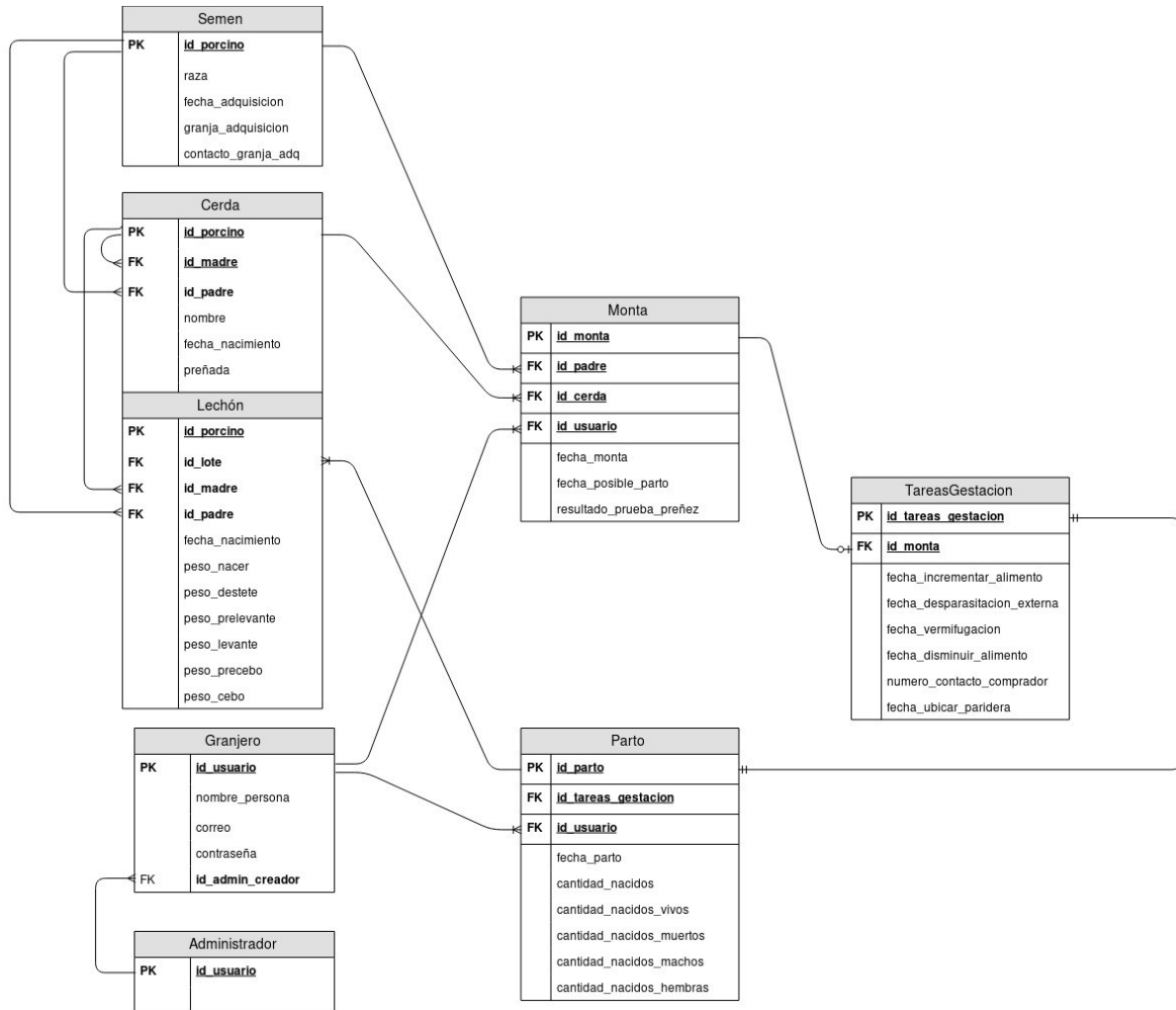
Figura 7. Diagrama de Bases de Datos
