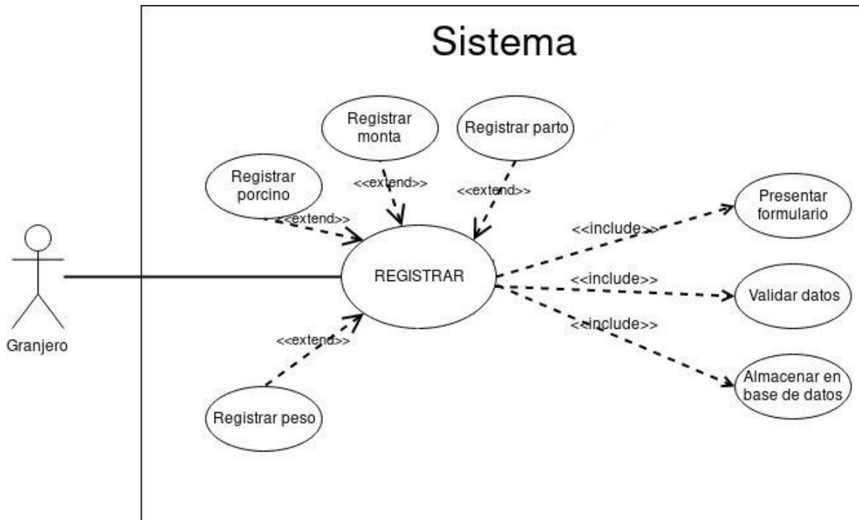
Figura 3. Diagrama de Casos de uso Registrar
