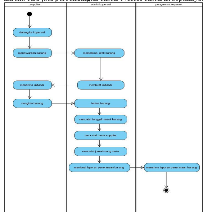
Gambar 1. Activity Diagram Sistem yang Berjalan
