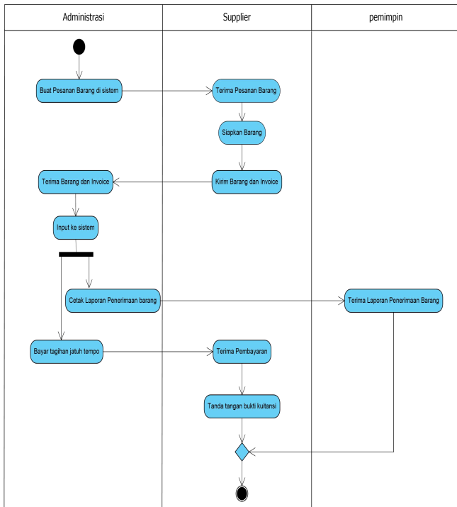
Gambar 3. Activity Diagram yang di usulkan
