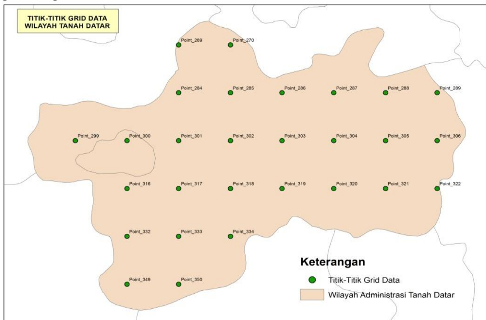
Gambar 1. Wilayah Tanah Datar dibagi menjadi titik-titik grid.
