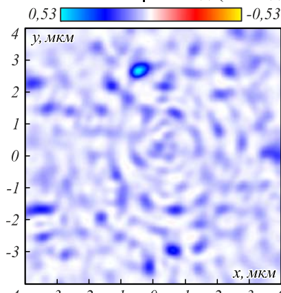
Рис. 9. Распределение проекции вектора Пойнтинга на оптическую ось S_z
