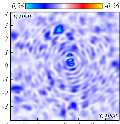
Рис. 8. Распределение интенсивности |E^2| на расстоянии 0,433 мкм от поверхности металлинзы (рис. 3)
