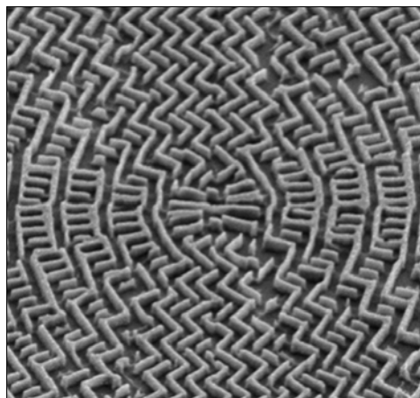
Рис. 3. Изображение изготовленной спиральной металинзы, полученное с помощью электронного микроскопа
