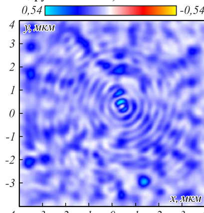
Рис. 10. Распределение интенсивности |E^2| на расстоянии 0,433 мкм от поверхности металлинзы
