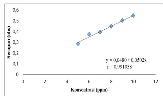
Gambar 1. Grafik Kurva Baku Kafein
