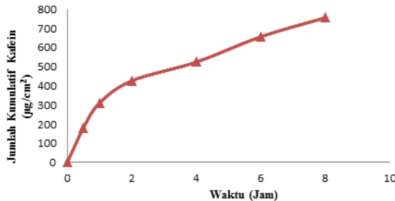
Gambar 4. Grafik Profil Jumlah Kumulatif Kafein Terpenetrasi Sediaan Gel-Krim
