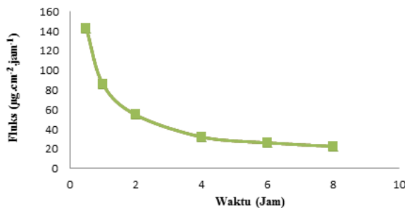
Gambar 6. Grafik Profil Fluks Kafein Sediaan Krim
