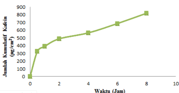
Gambar 2. Grafik Profil Jumlah Kumulatif Kafein Terpenetrasi Sediaan Gel
