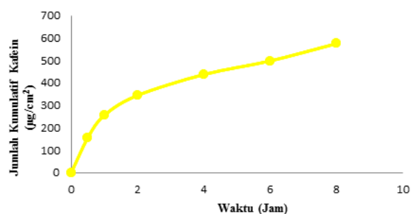
Gambar 3. Grafik Profil Jumlah Kumulatif Kafein Terpenetrasi Sediaan Krim
