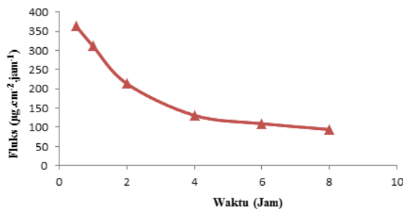
Gambar 7. Grafik Profil Fluks Kafein Sediaan Gel krim
