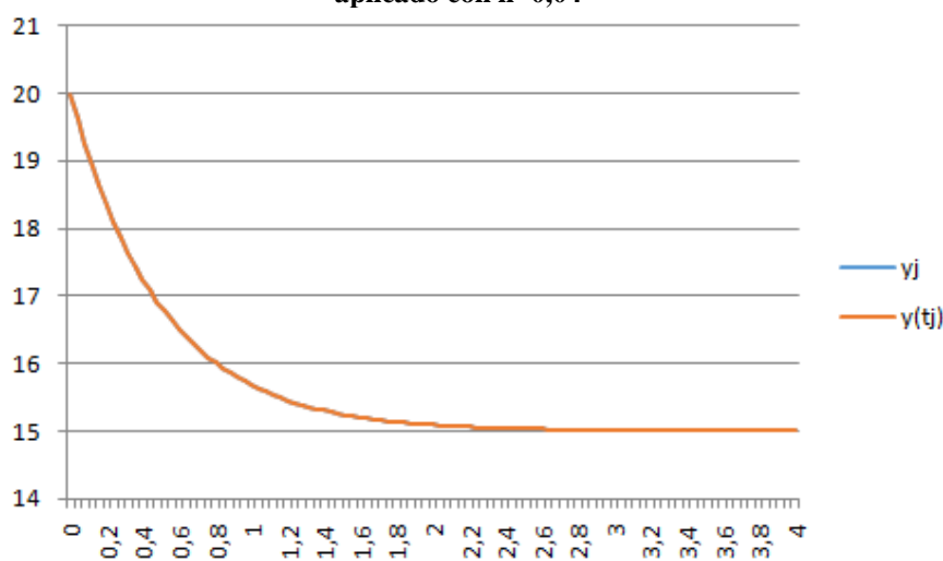
Figura 37. Aproximaciones y valor exacto para método de R-K de tercer orden mejorado aplicado con h=0,04
