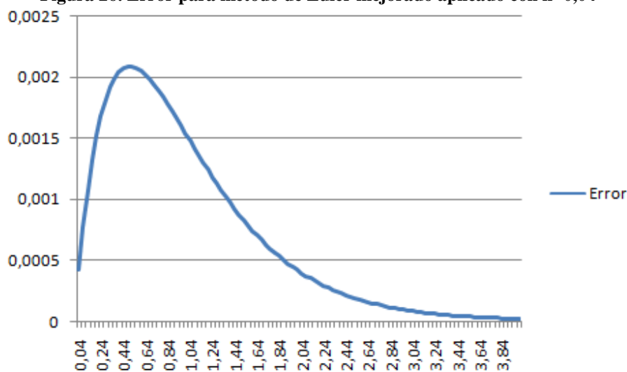
Figura 26. Error para método de Euler mejorado aplicado con h=0,04
