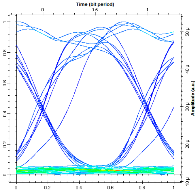
Figure 3: Eye Diagram of de-mod OOK signal-Uplink
