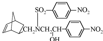
XVIIa
