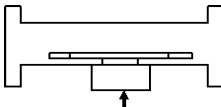
Рисунок 1. Хвильовідний фазоповертач.
