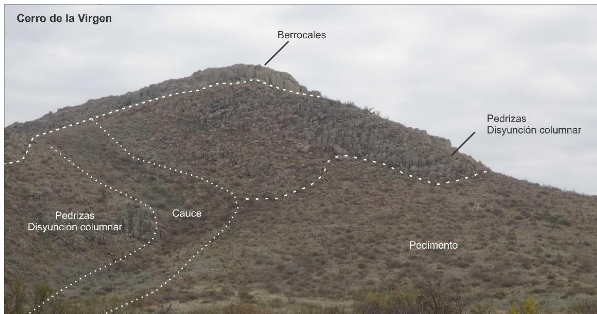
Figura 7.35. Geoformas y procesos geomorfológicos en el cerro de La Virgen. Fuente: elaborado por Duval.
