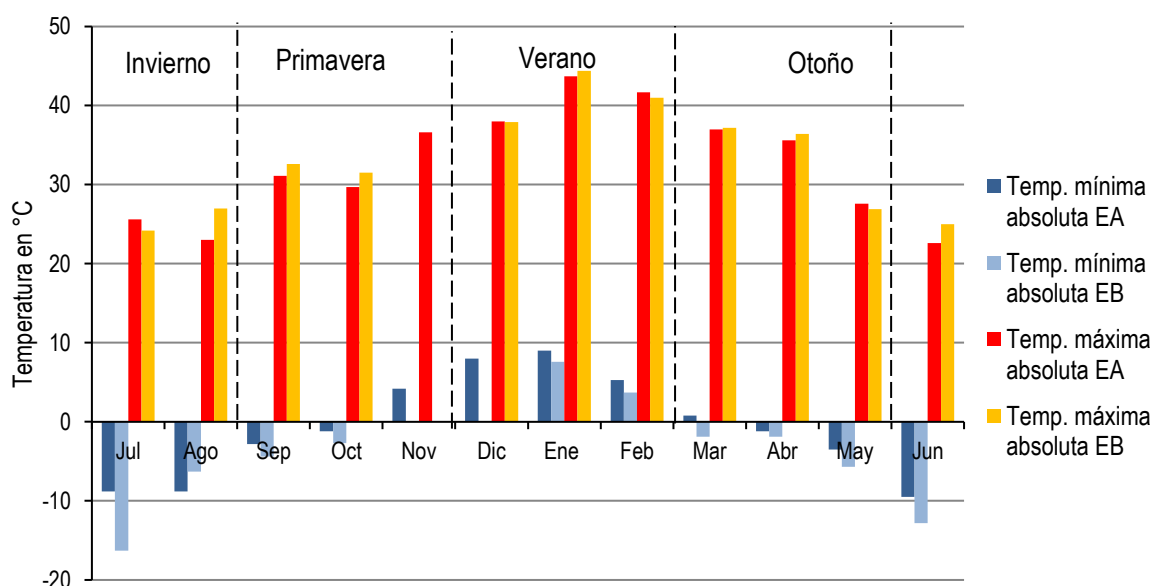
Figura 6.4. Distribución anual de las temperaturas absolutas en EA y EB para el año 2012. Fuente: elaborado por Duval.
