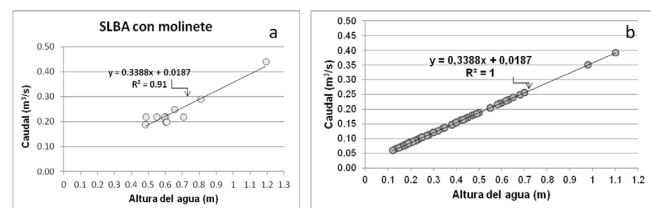
Figura 4 a. Medición del caudal con molinete. b. ajuste de todas las alturas del agua a la función.
