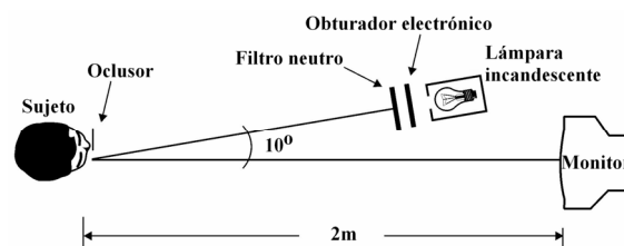
Fig. 1. Esquema del dispositivo experimental.
