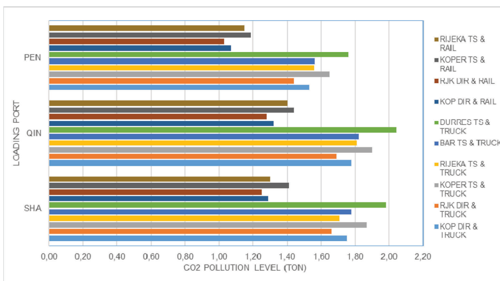
Figure 3 CO2 emissions between POL to Novi Sad (in tonnes) Slika 3. CO 2 emisije od luka ukrcaja do Novoga Sada (u tonama)
