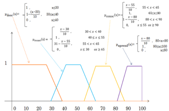
Fig. 2: definición de conjuntos difusos para los ítems atómicos (hojas del dominio)
