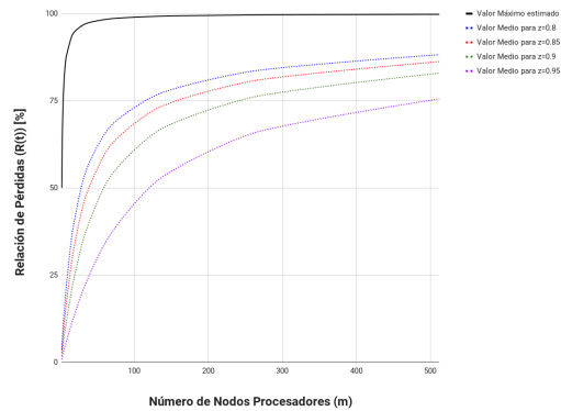
Figura 4. Relación de Pérdidas de cuadros Máxima y Media para Régimen Dinámico.
