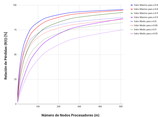
Figura 3. Relación de Pérdidas de cuadros Máxima y Media para Régimen Estático.
