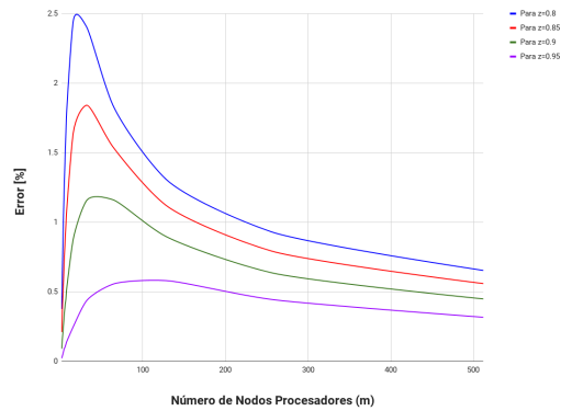
Figura 5. Diferencia entre la estimación de pérdida media de Régimen Dinámico y Estático.
