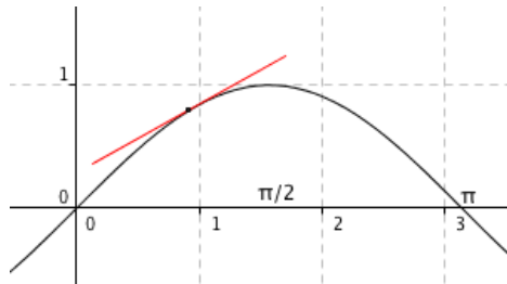
Figura 12. Tangente con pendiente de \sqrt{3}/3 en x = 0.95 .
