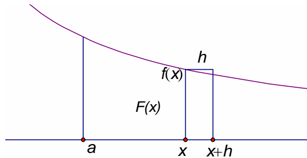
Figura 25. Incremento del área
