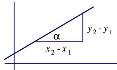
Figura 2. Pendiente de una recta.
