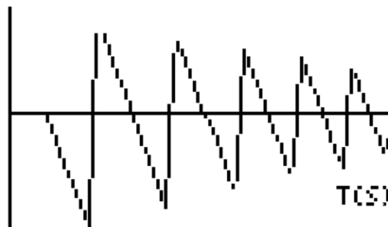
Figura 20. Velocidad de una pelota que rebota (Cory, 2010)
