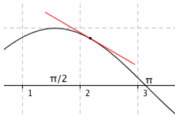
Figura 13. Tangente con pendiente -0.577 en x = 2.1 .
