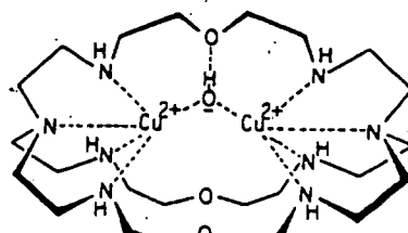
[(Cu_2(OH)L)^{3+}] (L = O-BISTREN)
