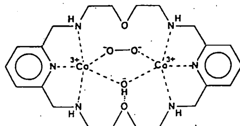
Co_2LO_2(OH)^{3+}
