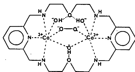
Co_2LO_2(OH)_3^+
