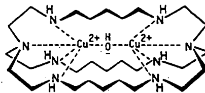
[(Cu_2(OH)L')^{3+}] (L' = C-BISTREN)
