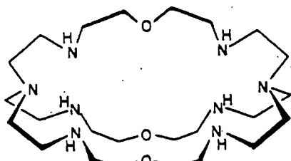
(O-BISTREN)
