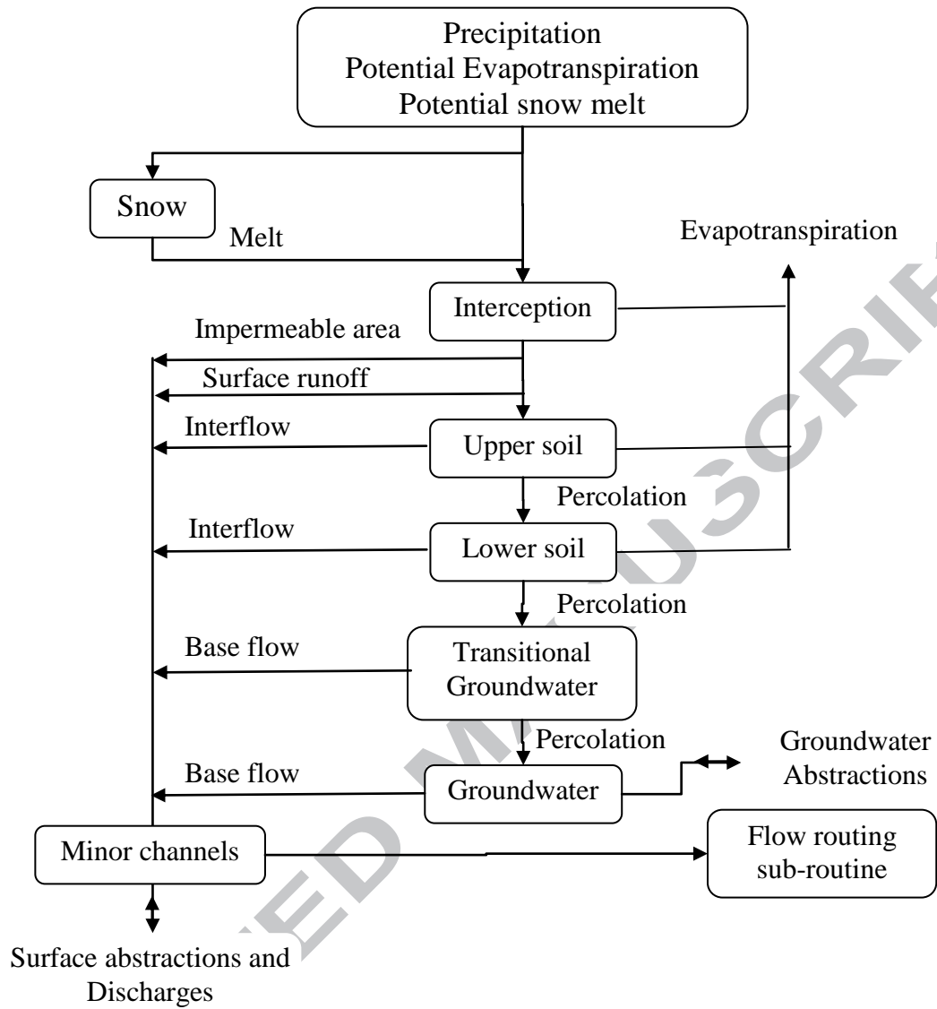
Fig. 3 HYSIM schematic
