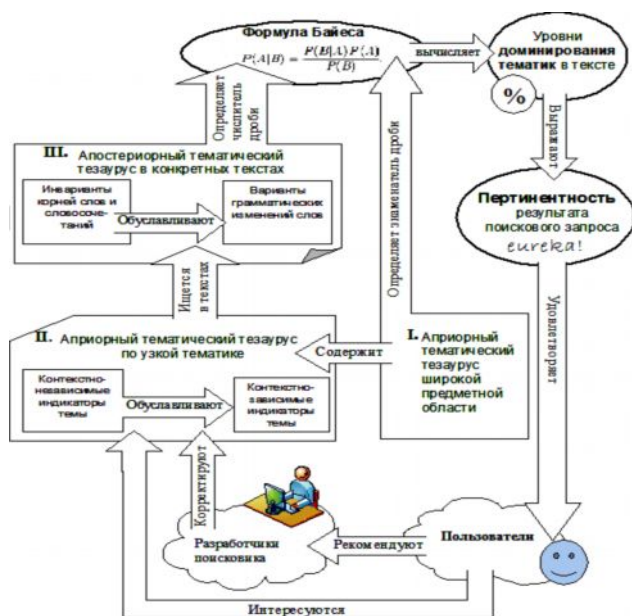
Рис. 4. Прикладная модель поисковой системы, основанной на pertinентности результатов запроса
