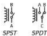
gambar 3 Konfigurasi Relay SPST dan Relay SPDT
