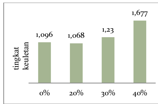
Gambar 6. Grafik nilai rata-rata uji impak
