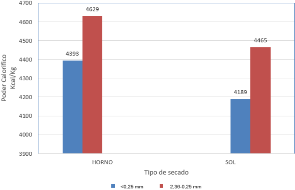
Gráfica 2 Poder calorífico de acuerdo a los pretratamientos
