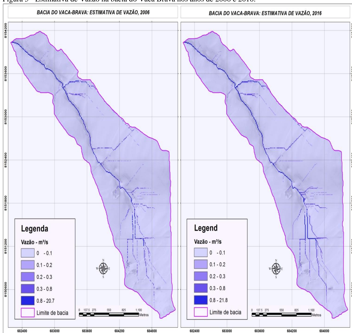
Figura 5 - Estimativa de Vazão na bacia do Vaca Brava nos anos de 2006 e 2016.
