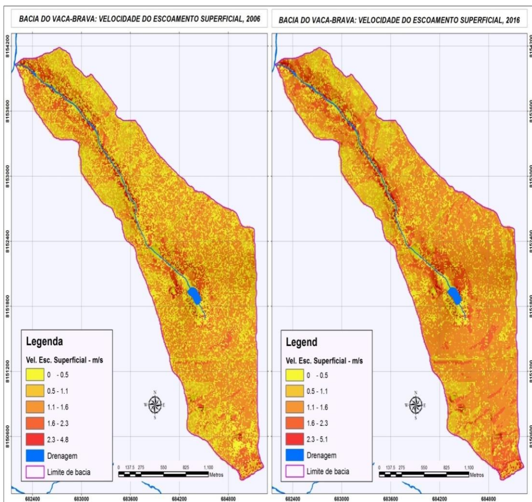
Figura 3 - Velocidade do escoamento superficial nos anos de 2006 e 2016.
