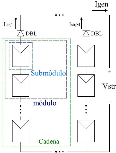
Figura 2. Composición de un generador fotovoltaico en configuración SP. Fuente: elaboración propia.
