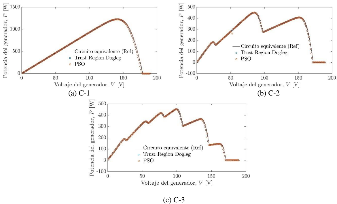
Figura 8. Curvas de Potencia vs Voltaje de un generador fotovoltaico formado por 15 submódulos, bajo las condiciones de irradiancia dadas en (a) C-1 (b) C-2 (c) C-3. Fuente: elaboración propia.
