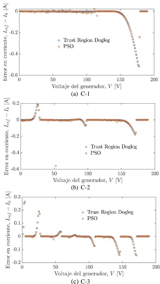
Figura 9. Error en corriente vs. Voltaje para un generador fotovoltaico formado por 15 submódulos en serie, bajo las condiciones de irradiancia dadas en (a) C-1 (b) C-2 (c) C-3. Fuente: elaboración propia.
