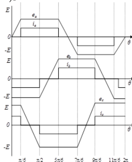
Gambar 3. Gelombang BEMF ( Back Electromotive Force ) dan Arus pada BLDC ( brushless DC ) [2]
