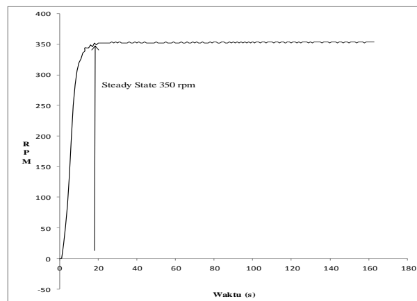
Gambar 12. Respon Kecepatan Motor Kondisi Close Loop
