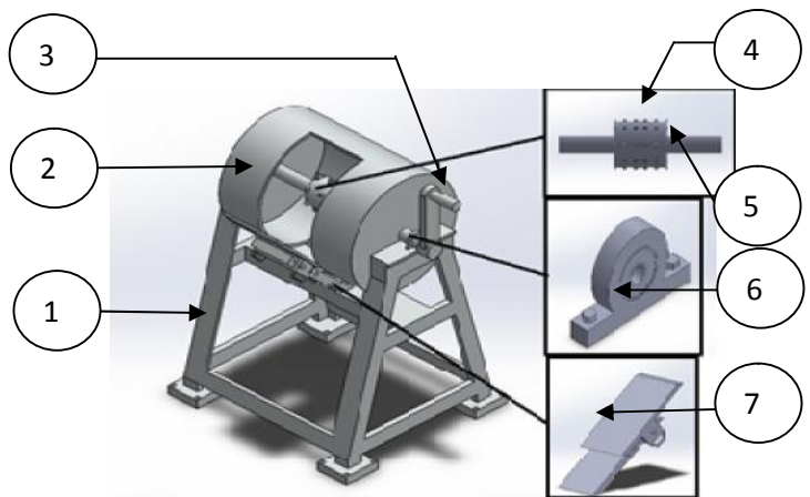
Gambar 3.2 Alat Pengurai Sabut
