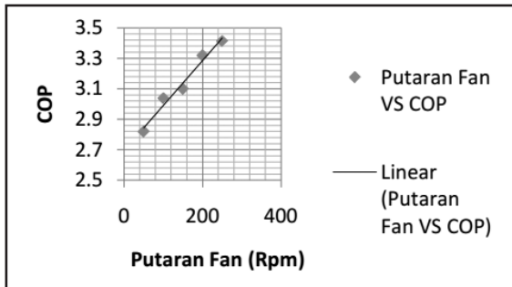
Gambar 4. Pengaruh kecepatan putar terhadap nilai COP.
