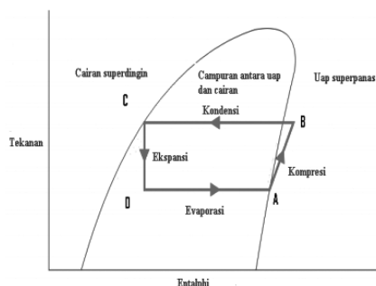
Gambar 2. Diagram P-h siklus kompresi uap
