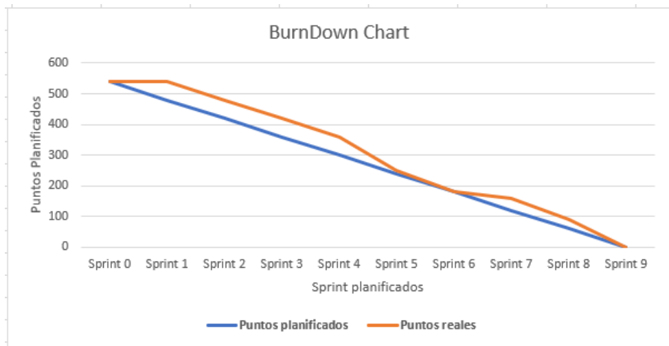
Gráfico 1-2: BurnDown Chart.
