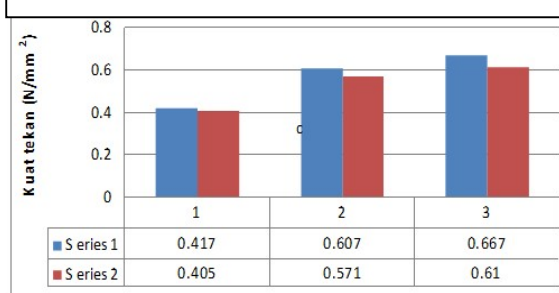
Gambar.2 Grafik perbandingan nilai kekuatan tekan
