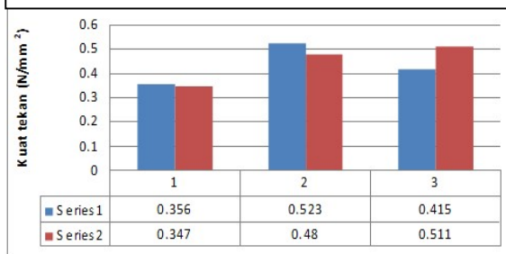
Gambar 3. Grafik perbandingan nilai kekuatan tekan
