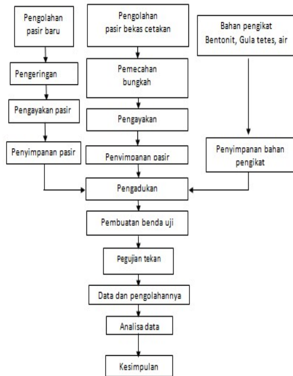
Gambar 1. Diagram alir pengaruh pasir cetak daur ulang dan pasir baru berpengikat waterglass terhadap cetakan
