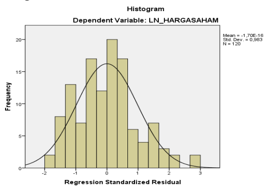
Gambar 1. Grafik Uji Normalitas Histogram (Setelah Transformasi)
