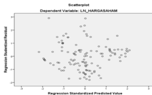
Gambar 3. Grafik Uji Heteroskedastisitas Scatterplot (Setelah Transformasi)
