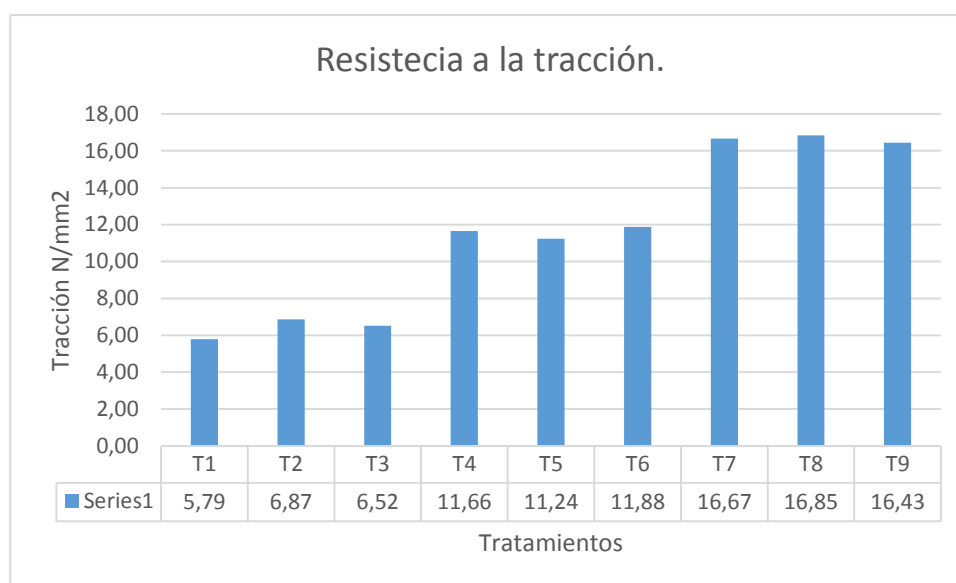
Figura 12. Comportamiento interacción de factores en resistencia a la tracción para cada uno de los tratamientos.
