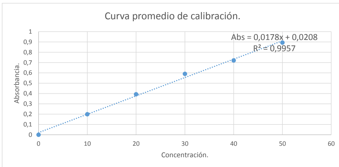
Figura 7. Curva promedio de calibración ácido gálico.
