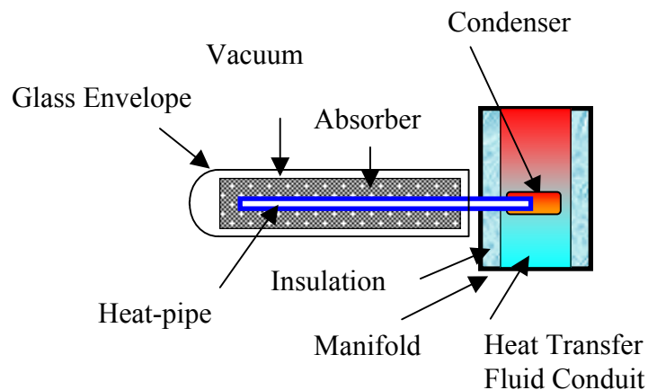
Fig. 1 Heat pipe ETSWH
