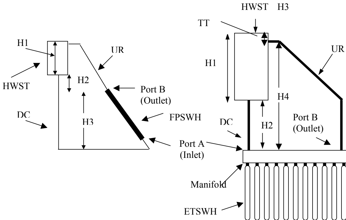
Fig. 2 Thermosyphon FPSWH
