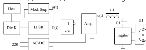
Рисунок 1. Запропонований пристрій
