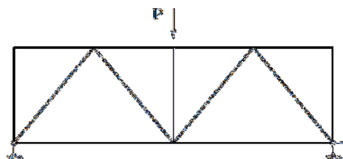
Рисунок 2. Схема закріплення та навантаження ферми
