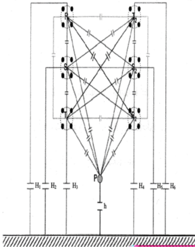
Gambar 7. Kapasitansi Pada Saluran Transmisi
