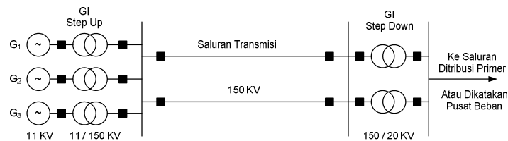
Gambar 6 : Diagram Satu Garis Sistem Saluran Transmisi
