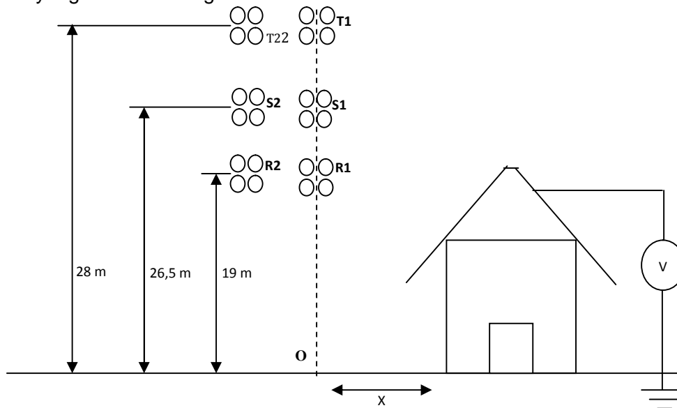
Gambar 12. Rangkaian Pengukuran Tegangan Induksi
