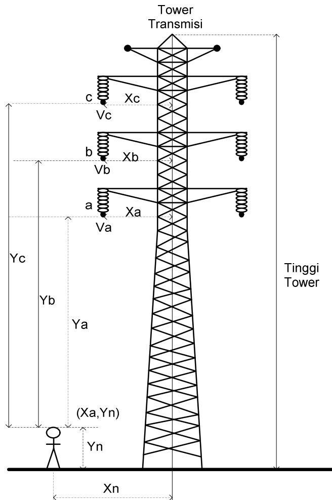
Gambar 11: Parameter Saluran Transmisi Tiga Fasa 150 KV Tanpa Dipengaruhi Oleh Objek Disekitarnya Dengan Titik Koordinat Manusia ( X_n & Y_n )
