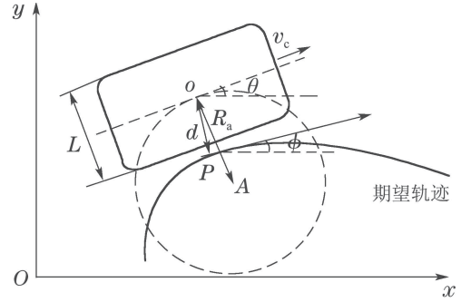
图1 运动学模型
