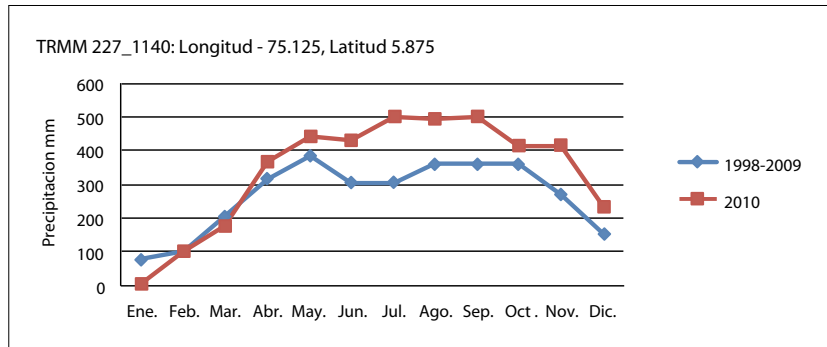
Figura 5. Alteraciones en la precipitación en el 2010 en una estación satelital de la cuenca del río Porce.
