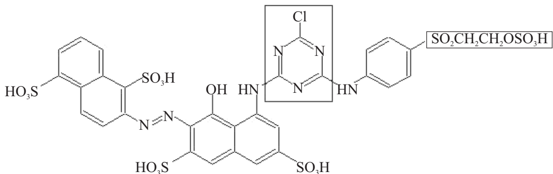
Figura 2 Estructura química del colorante Rojo Brillante Remazol 3BS [22]
