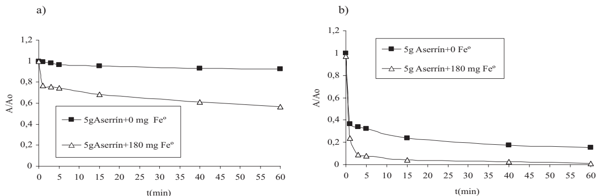
Figura 4 Variación de la absorbancia normalizada versus el tiempo para diferentes cantidades de ZVI a) pH= 5,2, 5 g de aserrín pretratado con formaldehído al 1%, concentración de colorante = 70 mg/L, volumen de solución = 60 ml. b) pH= 2,0, 5 g de aserrín pretratado con formaldehído al 1%, concentración de colorante = 70 mg/L, volumen de solución = 60 ml
