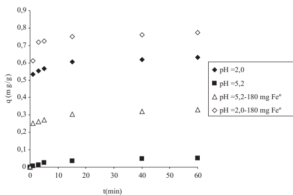
Figura 3 Efecto del pH y la cantidad de partículas ZVI en la adsorción del RR239
