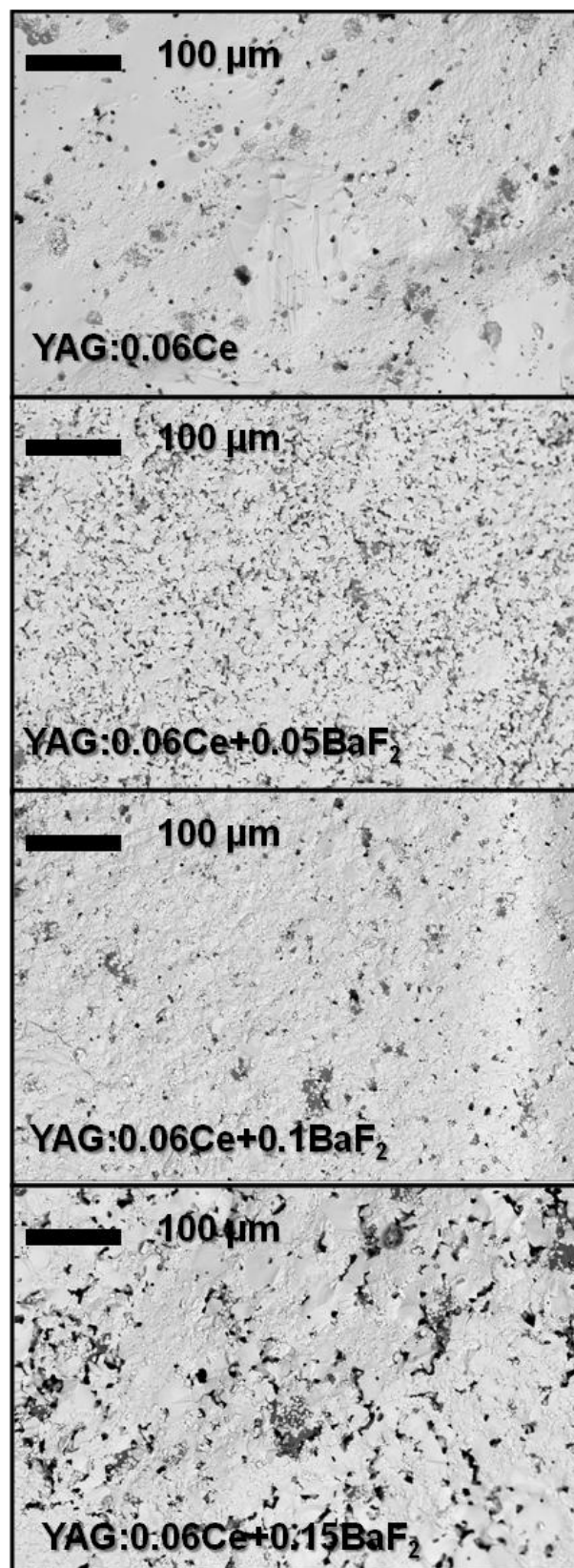
Fig. 3. SEM micro-images.
