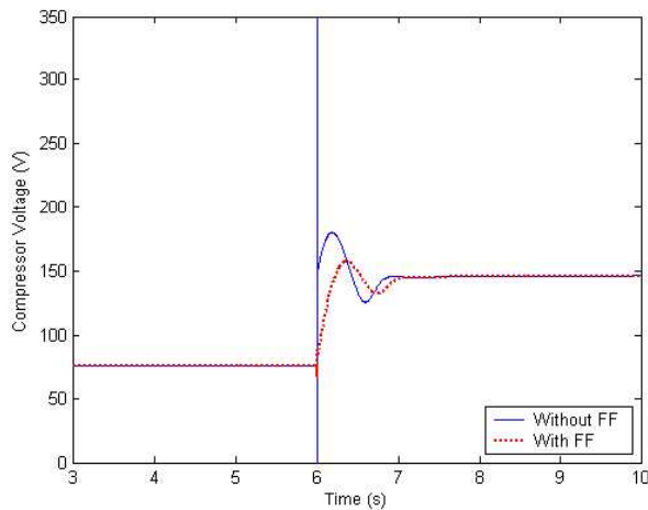
Figura 17: Voltaje del compresor generado por un GPC con y sin efecto Feedforward.
