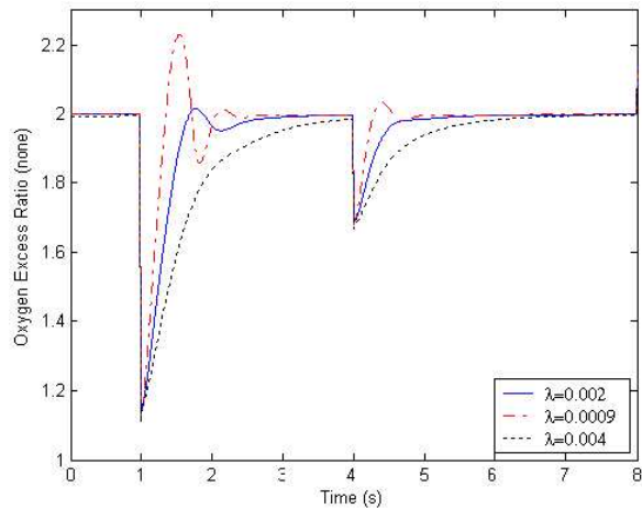
Figura 8: Control del exceso de oxígeno mediante un GPC sintonizado con diferentes pesos de control en simulación dinámica variando la corriente.
