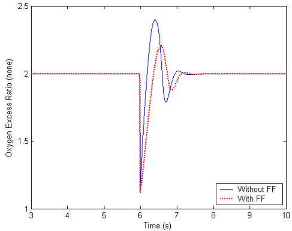
Figura 16: Exceso de oxígeno controlado por GPC con y sin efecto Feedforward.
