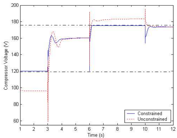
Figura 11: El voltaje del compresor generado por un GPC con y sin restricciones
