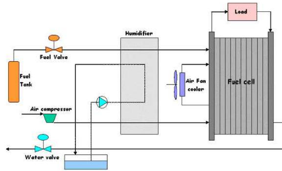
Figura 1: Esquema de los actuadores de la pila de combustible y de los equipos auxiliares.
