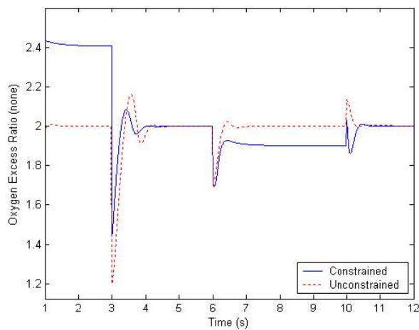
Figura 10: Control del exceso de oxígeno mediante un GPC con y sin restricciones.
