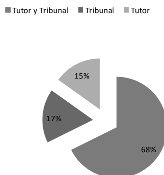
ILUSTRACIÓN 1: AGENTES EVALUADORES
