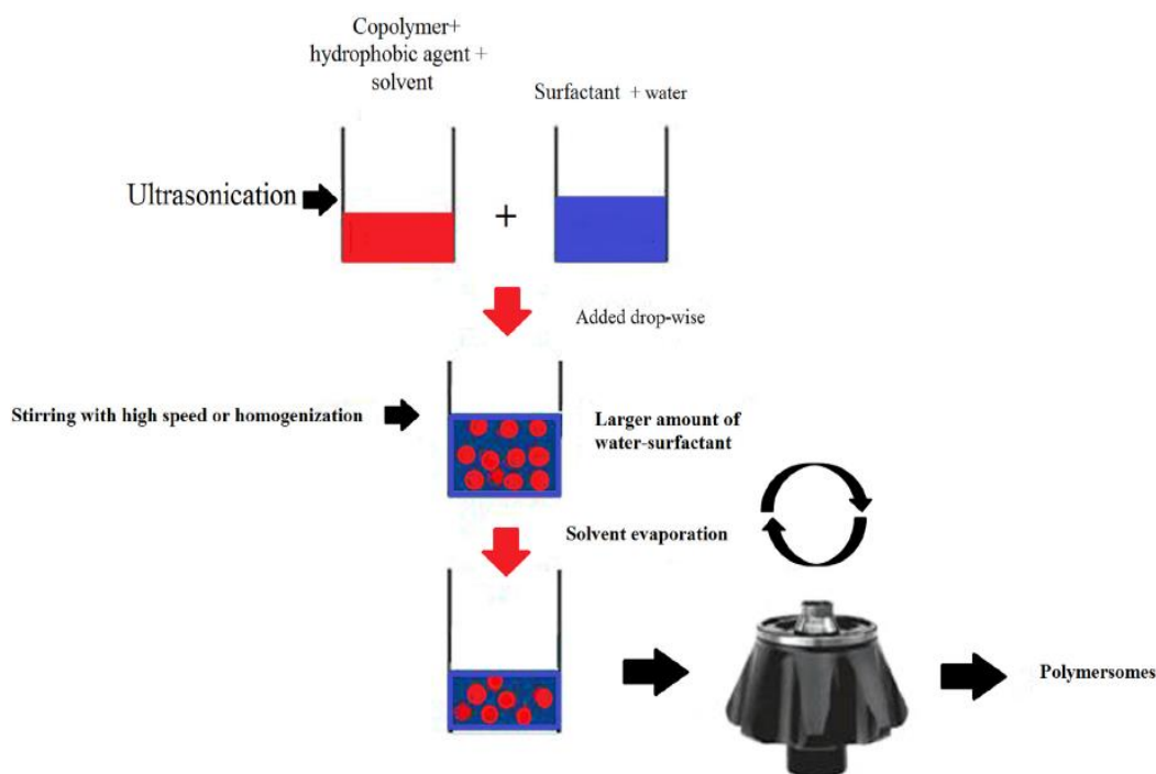
Figura 6. Representación esquemática de la elaboración de polimersomas mediante la técnica de doble emulsión por extracción- evaporación del solvente (Mohammadi et al., 2017).
