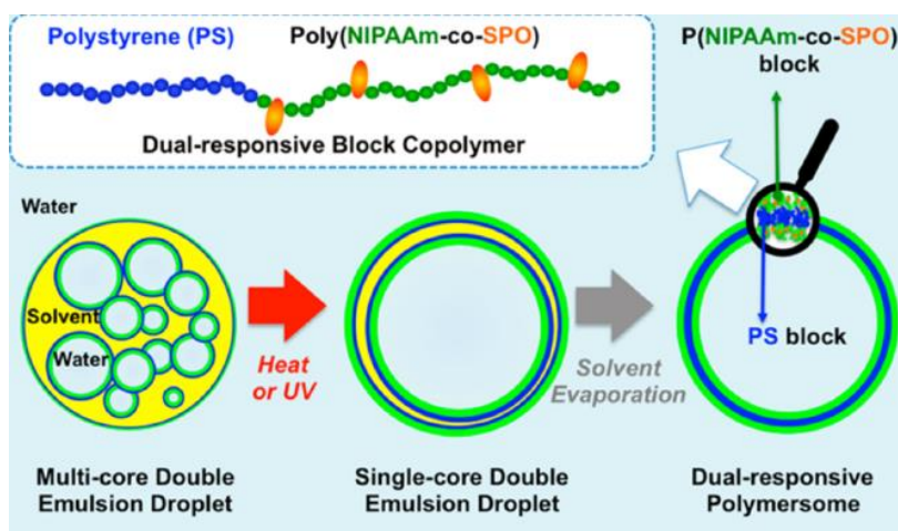
Figura 7. Representación esquemática de la formación de polimersomas mediante el empleo de estímulos (Mohammadi et al., 2017).
