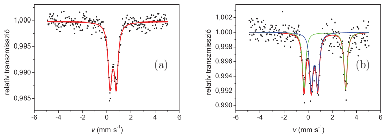
16. ábra. A \text{Fe}(\text{NO}_3)_3 \cdot 9\text{H}_2\text{O} és IAA összekeverésével kapott minták Mössbauer-spektrumai 20 perc elteltével fagyaszta (a) abszolút etanolban és (b) etanol-víz 1:1 térfogatarányú elegyében. A Fe:IAA arány mindkét esetben 1:3 volt.
