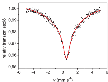
9. ábra. A 0,1 M-os ^{57}\text{Fe}(\text{NO}_3)_3 oldat Mössbauer-spektruma 80 K hőmérsékleten (pH~1).
