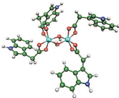
21. ábra. Az [(IA)_2Fe(OH)_2Fe(IA)_2] komplex sematikus szerkezete gömb és pálcika modell segítségével ábrázolva.
