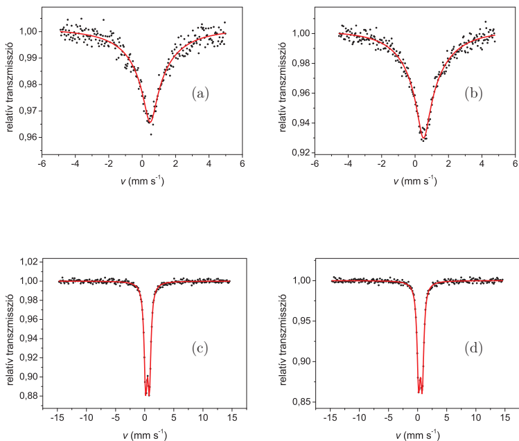
37. ábra. (a) A kiindulási 0,1 \text{ M } ^{57}\text{FeCl}_3 , (b, c, d) és a belőle készített 0,05 \text{ M } ^{57}\text{Fe}^{\text{III}} -citrát oldatok Mössbauer-spektrumai 80 \text{ K} hőmérsékleten. A ^{57}\text{FeCl}_3 oldat pH-ja (a) 1,3 ; a ^{57}\text{Fe}^{\text{III}} -citrát oldatok pH-ja (b) 1,2 ; (c) 4,0 és (d) 5,9 voltak.
