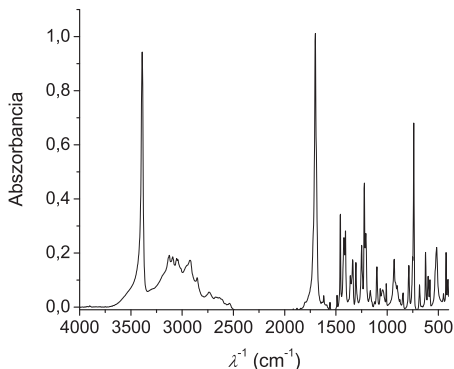
18. ábra. A szilárd indol-3-ecetsav IR spektruma.
