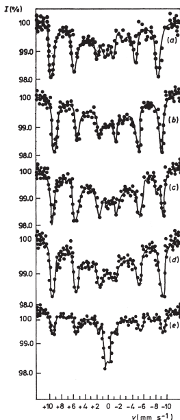
8. ábra. 0,05 M-os \text{Fe}(\text{NO}_3)_3 oldatok spektrumai 4,2 K-en: (a) 65%-os \text{HNO}_3 , (b) 30%-os \text{HNO}_3 , (c) 11,2%-os \text{HNO}_3 , (d) \text{pH}=1,0 , (e) \text{pH}=2,0 [30] alapján.
