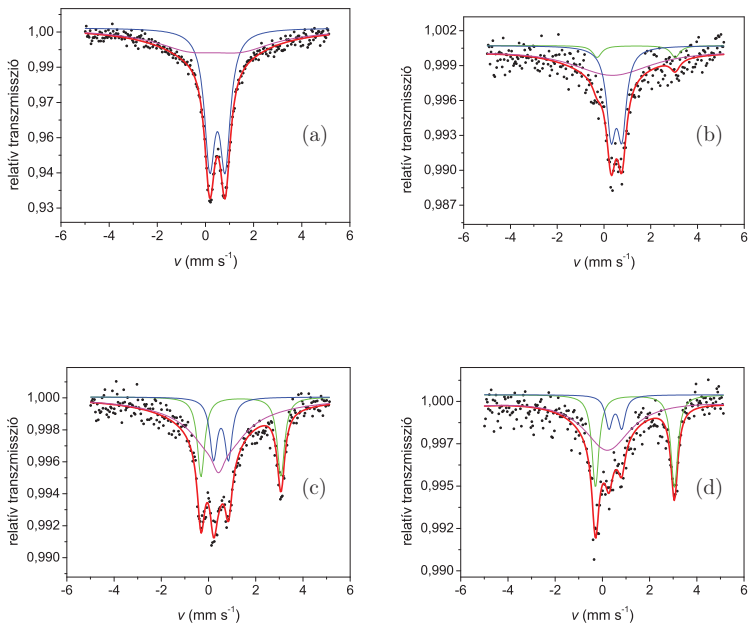
25. ábra. Az IAA tartalmú oldatokkal azonos körülmények között készített (a) \text{Fe}^{3+} -TRP, (b) \text{Fe}^{3+} -ICA, (c) \text{Fe}^{3+} -IPA, és (d) \text{Fe}^{3+} -IBA oldatok Mössbauer-spektrumai 80 K hőmérsékleten, 15 perc állás után fagyasztva.
