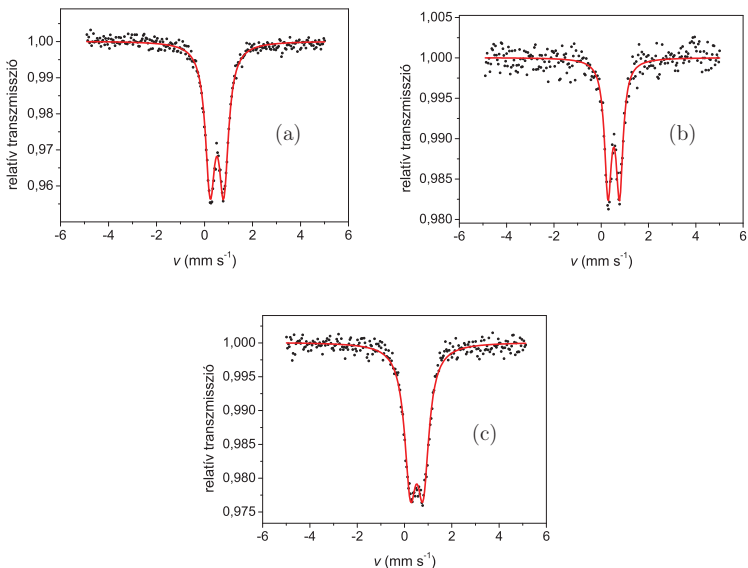
17. ábra. (a) A szilárd Fe-IAA komplex és annak (b) abszolút etanol, (c) aceton oldószerekben készített oldatainak Mössbauer-spektrumai 20 perc elteltével fagyaszta.
