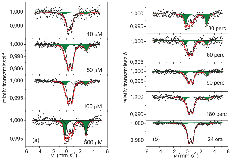
43. ábra. Vashiányosan nevelt, majd \text{Fe}^{\text{III}} -citráttal elátott uborka gyökerek Mössbauer-spektrumai 80 \text{ K} hőmérsékleten: (a) 30 perc vasellátási idő, növekvő Fe-koncentráció (b) 500 \mu\text{M} Fe-koncentráció, növekvő vasellátási idő.
