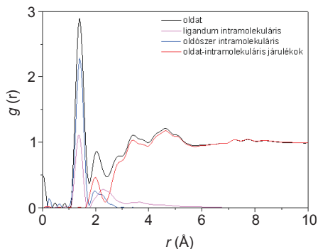
20. ábra. A [(IA)_2Fe(OH)_2Fe(IA)_2] 0.5 M-os metanolos oldatában mért párkorrelációs függvény és a számolt oldószer intramolekuláris, ligandum intramolekuláris járulékok, továbbá a különbség = (oldat)–(intramolekuláris járulékok az oldószerből és a ligandumból) párkorrelációs függvény. A modellalkotás és az illesztés a különbséggörbére lett végezve.
