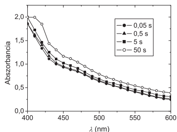
14. ábra. Abszolút etanolban oldott szilárd Fe-IAA komplex látható tartományban felvett spektruma vízzel való elegyítés után, az eltelt idő függvényében.
