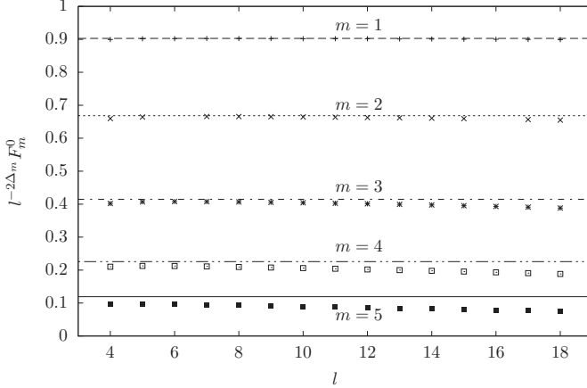
1.6. ábra. Vertexoperátorok vákuum-várhatóértékei
