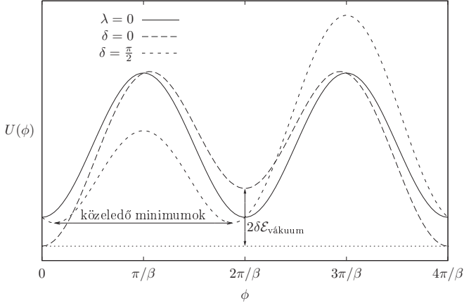
2.1. ábra. Az n = 2, m = 1 potenciál
