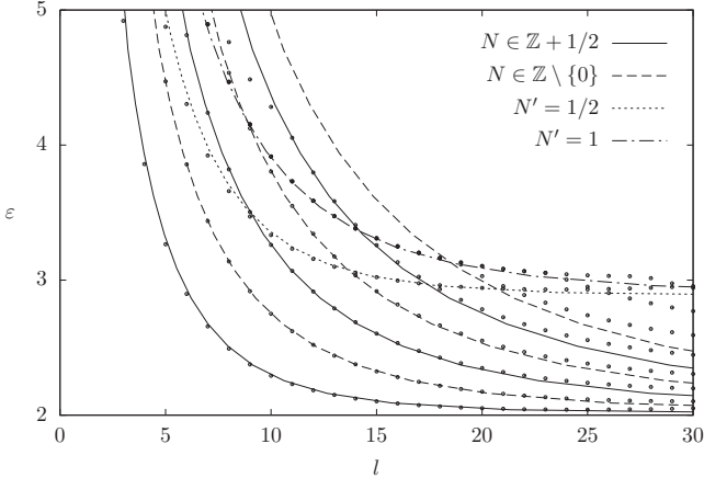
1.4. ábra. Kétkink-állapotok
