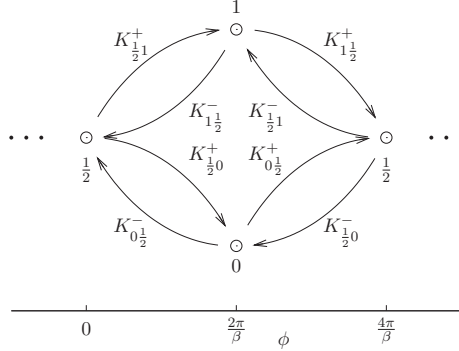
3.3. ábra. A szuperszimmetrikus sine–Gordon-modell kinkjeinek szomszédási diagramja
