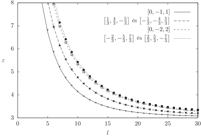
1.5. ábra. Háromkink-állapotok
