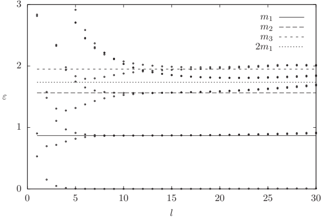
1.2. ábra. Lélegzőtömegek a 2-csavart modellben ( p = \frac{2}{7} , s = 0 , q = 0 )
