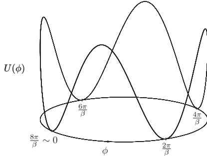
1.1. ábra. A negyedik minimumánál azonosított potenciál
