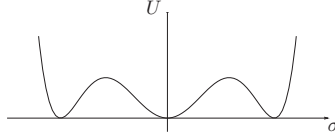
2.9. ábra. Az RSOS 3 modell vákuumszerkezet e
