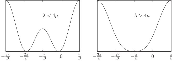
2.10. ábra. Másodrendű fázisátmenet a klasszikus potenciálban
