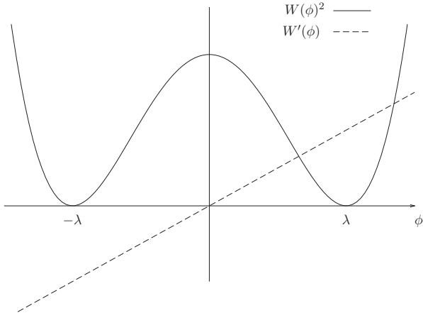
3.2. ábra. A szuperszimmetrikus Landau–Ginzburg-potenciál
