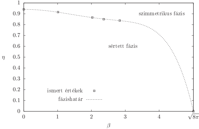
2.14. ábra. Fázisdiagram
