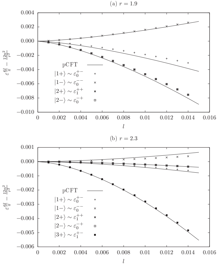
3.4. ábra. TCSA- és pCFT-energiaszintek összevetése
