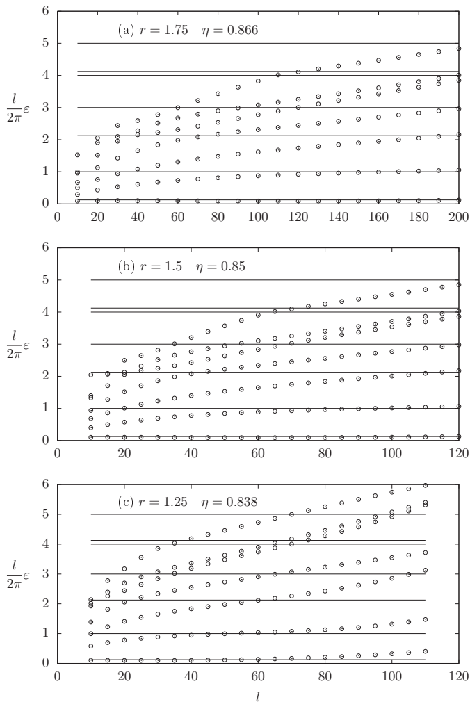
2.13. ábra. Kritikus TCSA-spektrumok
