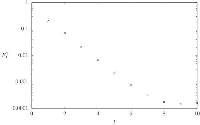
1.7. ábra. F_1^1(l) exponenciális lecsengése
