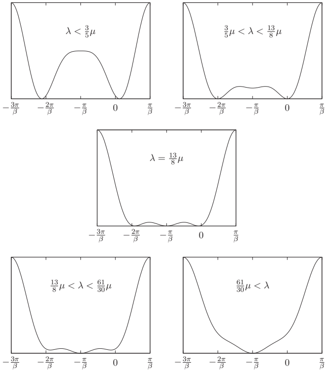
2.11. ábra. Elsődrendű fázisátmenet a potenciálban \kappa = -2/5\mu és \nu = 0 mellett
