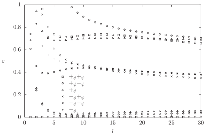
3.5. ábra. Az IR TCSA-spektrum alsó állapotai ( r = 3.05 )
