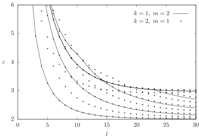
1.3. ábra. Hiányzó antiszimmetrikus állapotok ( p = \frac{2}{7} , s = 0 )
