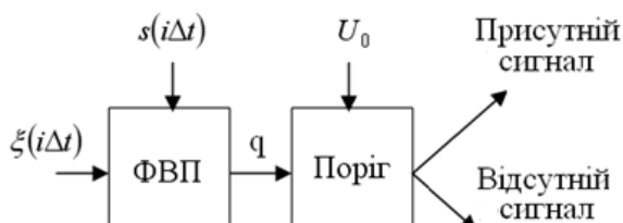
Рисунок 1. Структурна схема виявлення сигналу у суміші із завадами
