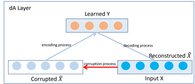
Fig. 4: The Denoising Autoencoder Layer
