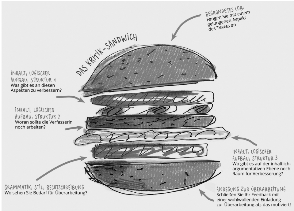
Abb. 1: Kritik-Sandwich
