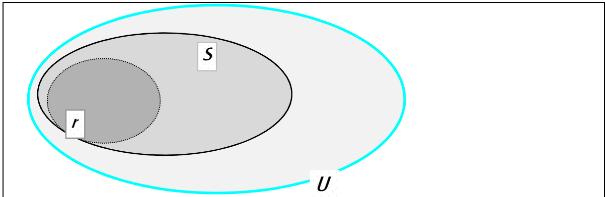
Abbildung . Responsemenge r , Stichprobe S , Population U mit r \subset S \subset U .
