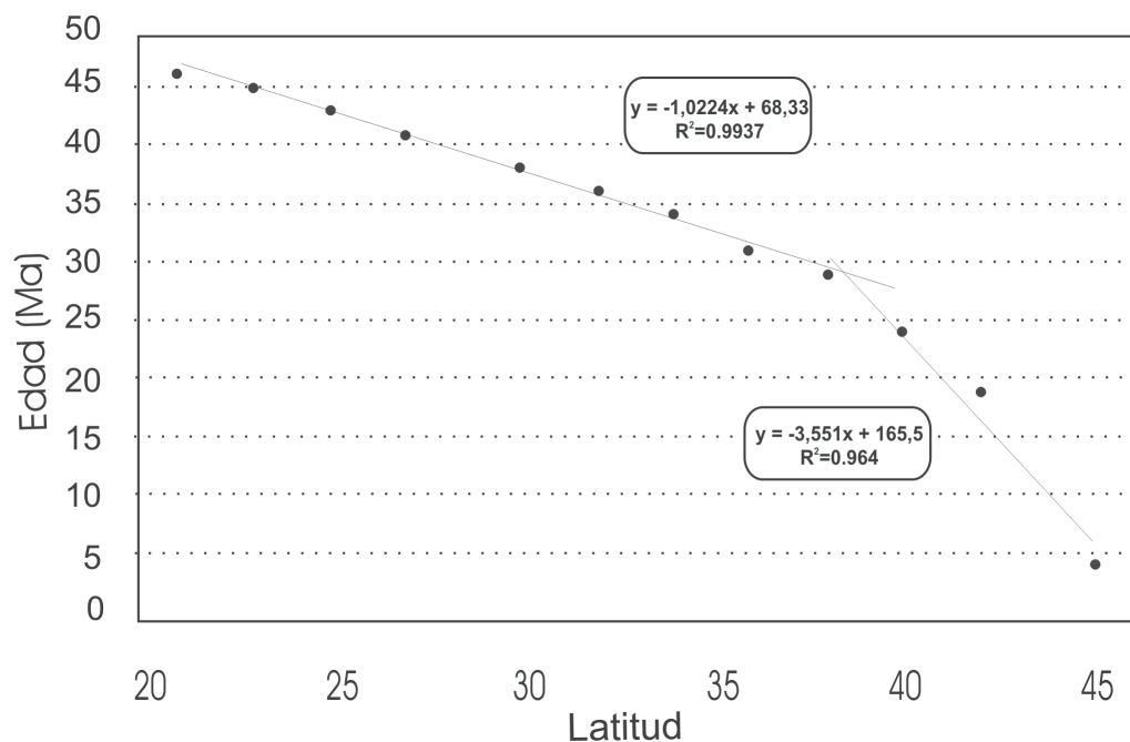
Figura 5: Edad de fondo oceánico en función de la latitud (Cuadro 1).
