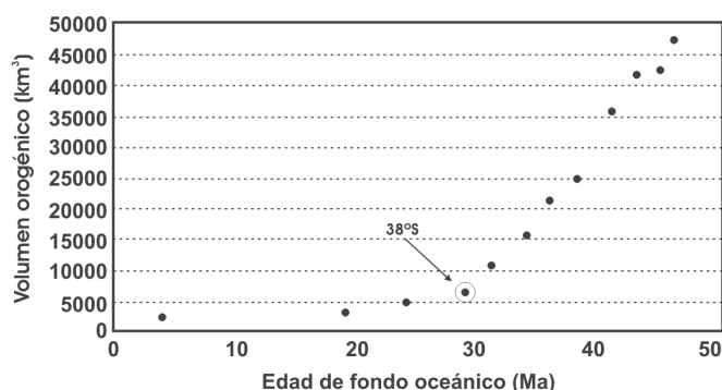
Figura 6: Variación del volumen orogénico en el sector de estudio de acuerdo a la edad de losas oceánicas subducidas.
