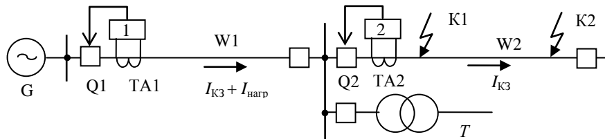
Рис. 2. Фрагмент сети, защиты которой требуют согласования характеристик
